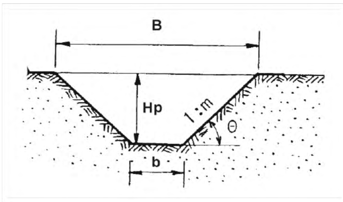
Слика 18: Изглед профила канала
