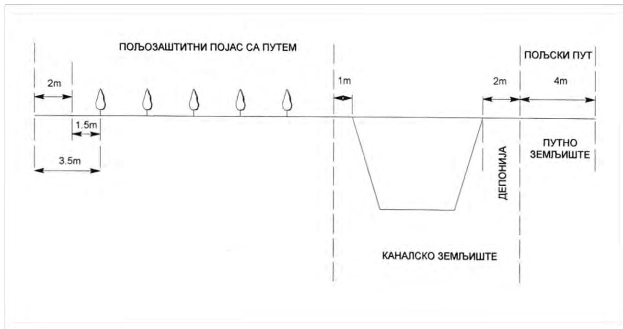
Слика 19: Пример профила пољозащитног појаса са пољским путем и каналом
