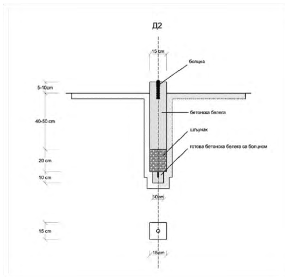
Слика 20: Изглед и димензије белеге ТИП Д2 са подземним центром
