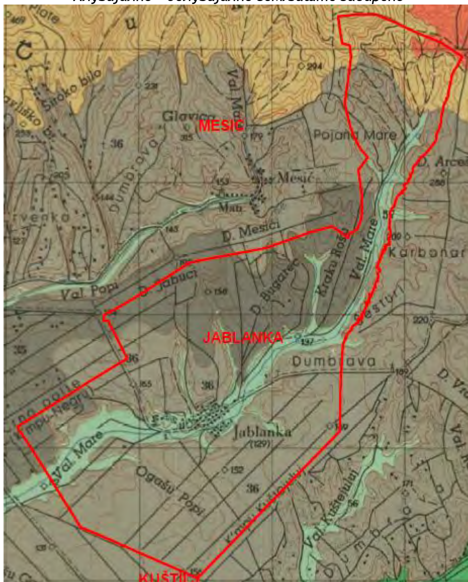
Слика 7: Педолошка карта КО Сочица 1
