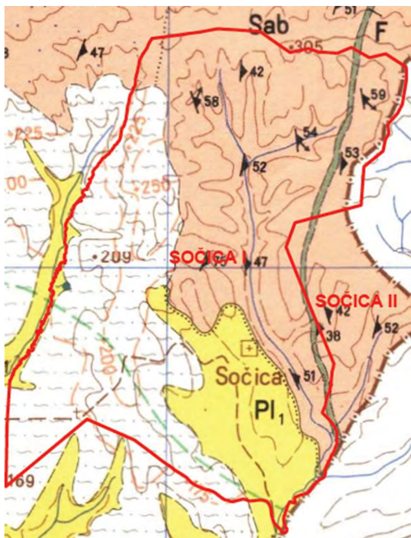
Слика 4: Геолошка карта КО Сочица 1
